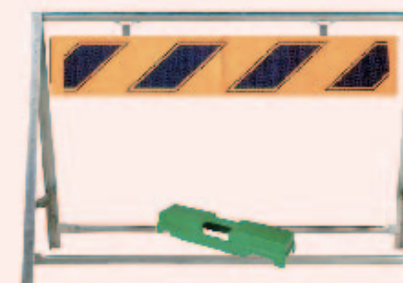
メッキA型バリケード (160) 高さ800×幅1200mm 約6.6kg 坂ターボリン仕様
